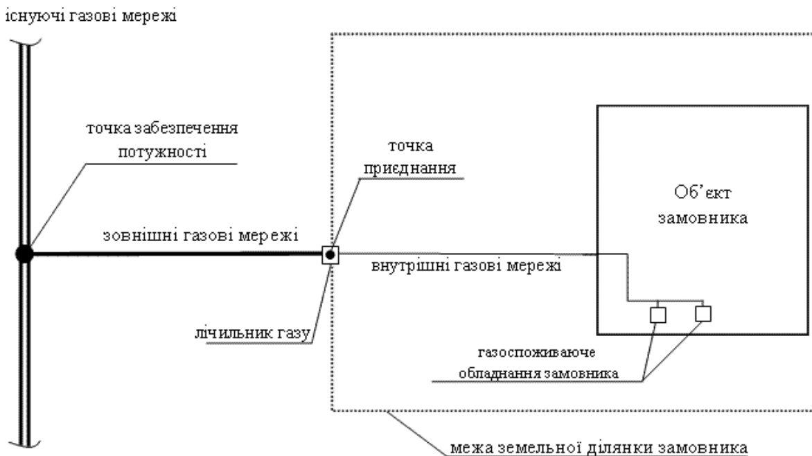
Рис. Принципова схема приєднання
